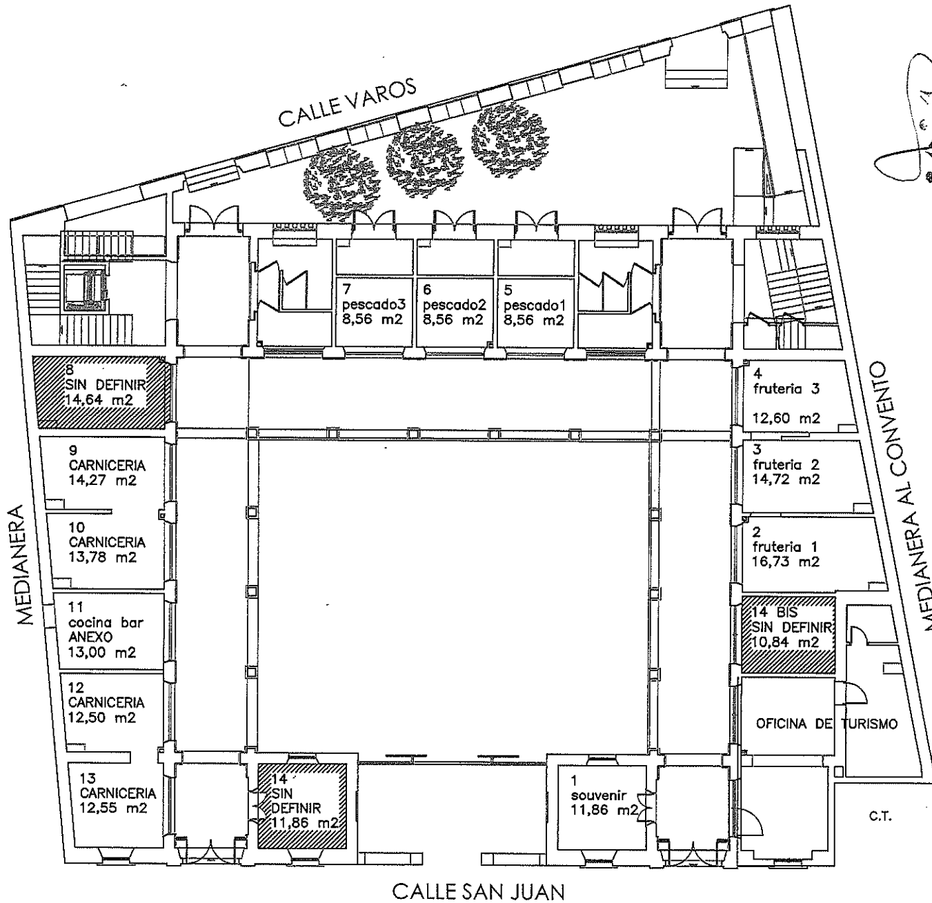
PLANTA BAJA
